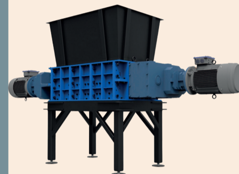
ДВОВАЛКОВА ДРОБАРКА RF-420
